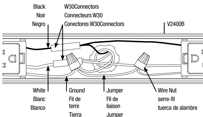
FIG. 2B WIRE NUT METHOD IMAGE 2B MÉTHODE DU CAPUCHON DE CONNEXION FIG. 2B MÉTODO CON CONECTOR DE RESORTE
