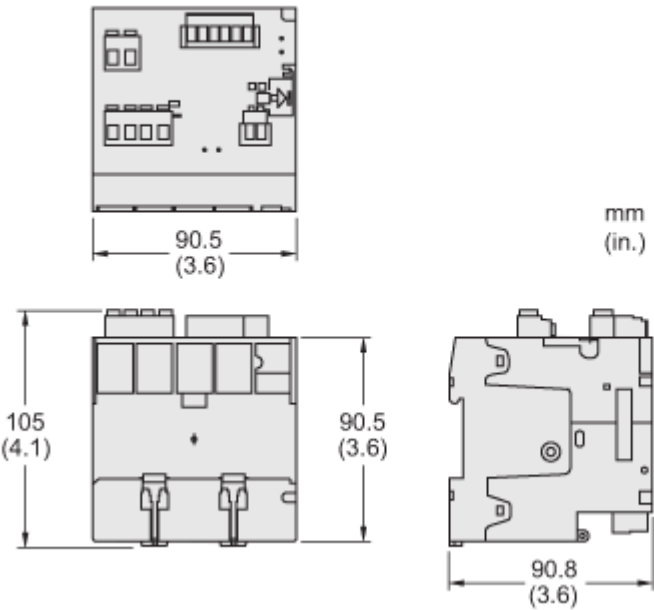
PM8000 DIN Rail Mount Meter
