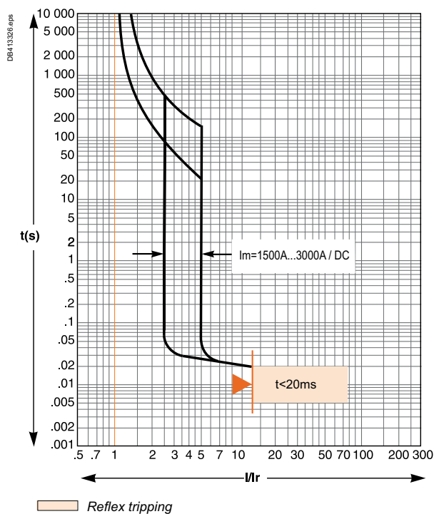
L-Frame 800A
