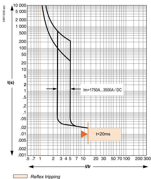
L-Frame 700A
