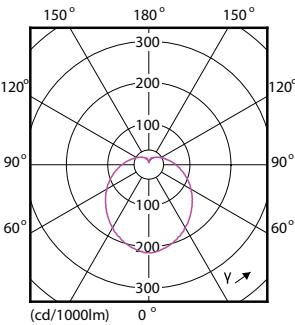
Light Distribution Diagram - 9A19/CNG/830/FR/P/E26/ND 4/1CT
