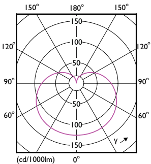
Light Distribution Diagram - 14A19/CNG/840/FR/P/E26/D 12/1CT
