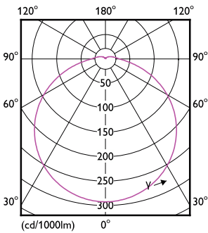
Light Distribution Diagram - 16UFO/PER/865/FR/P/E26/ND 4/1PF
