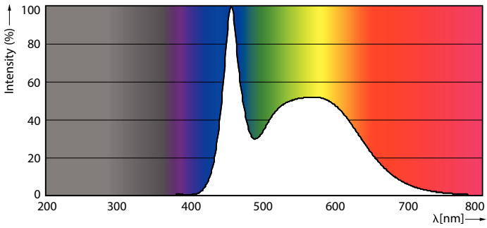
Spectral Power Distribution Colour - 16UFO/PER/865/FR/P/E26/ND 4/1PF
