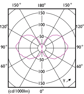
LEDbulb BA11 4,5W E12 820 Amber
